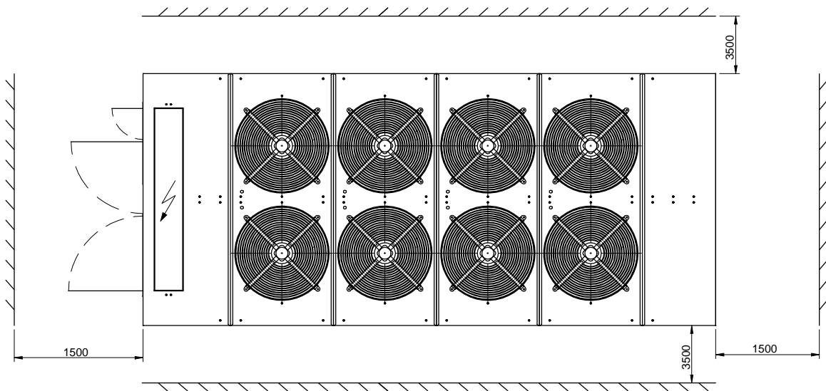
VISTA DALL'ALTO TOP VIEW
