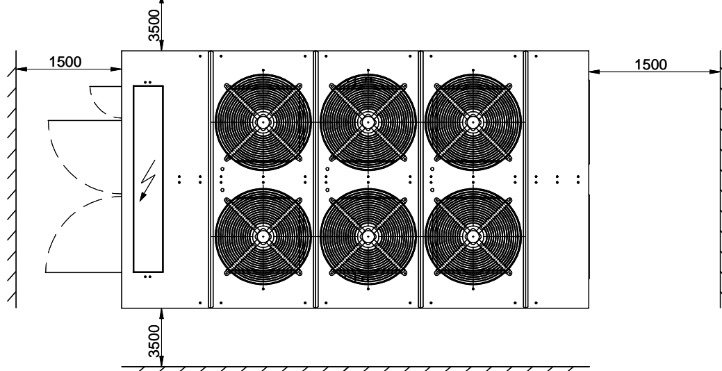
VISTA DALL'ALTO TOP VIEW
