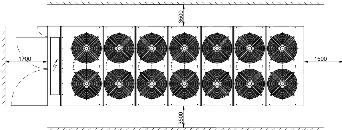
VISTA DALL'ALTO TOP VIEW
