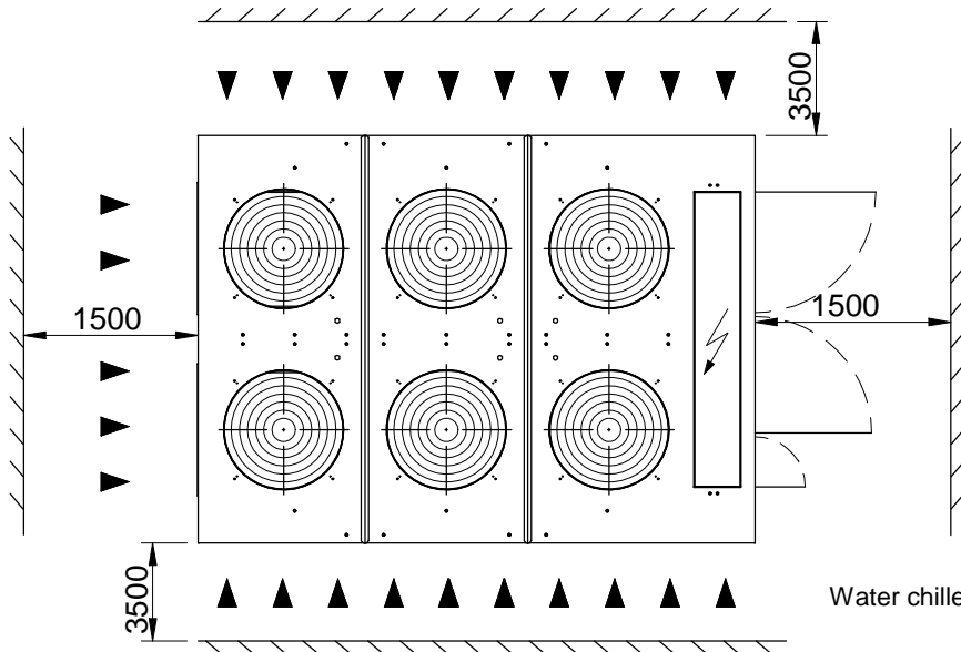
VISTA DALL'ALTO TOP VIEW
