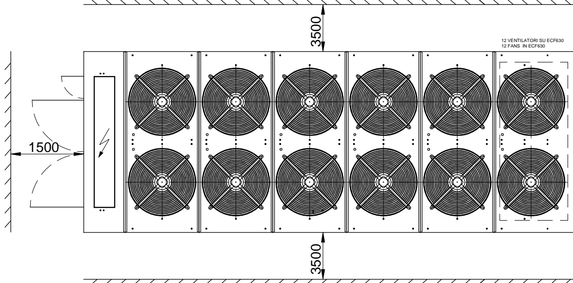
VISTA DALL'ALTO TOP VIEW
