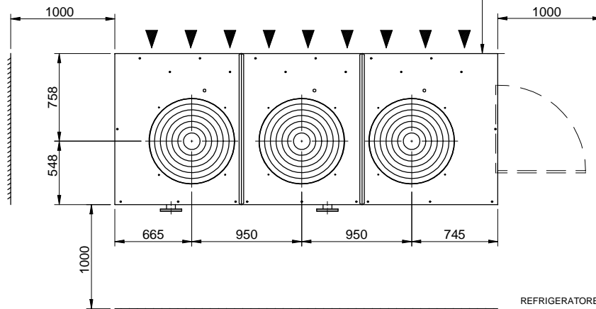
VISTA DALL'ALTO TOP VIEW
